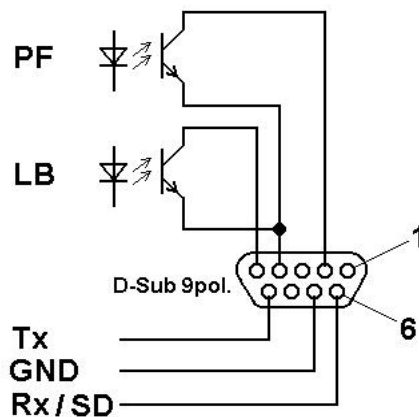
Abb. 6: USV interne Beschaltung der Kommunikations- Schnittstelle
