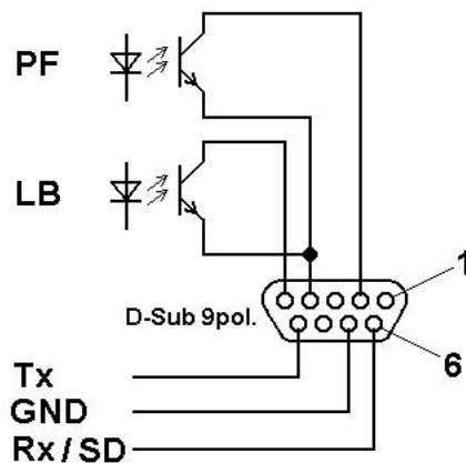
Abb. 6: USV interne Beschaltung der Kommunikations- Schnittstelle
